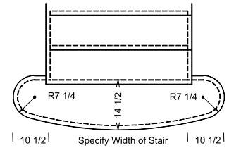
JP-8015-BOW
