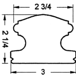
JP-6140
