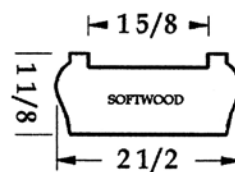
JP-6046
