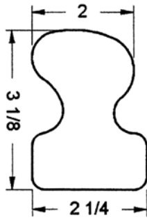
JP-6139
