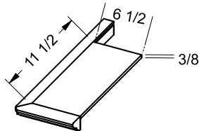
JP-8071 6.5
