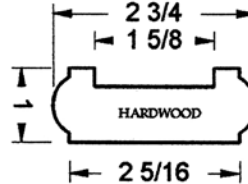
JP-6047
