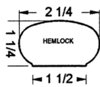
JP-6042
