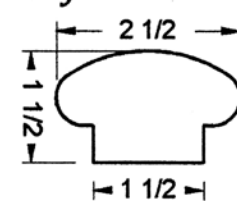
JP-6152
