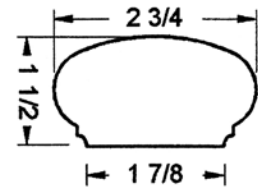
JP-6147
