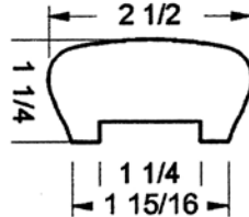
JP-6243
